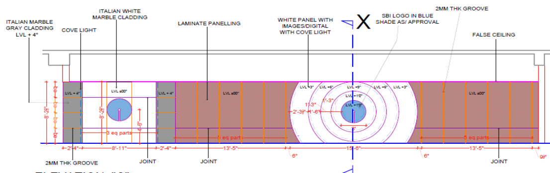
ELEVATION "C"
